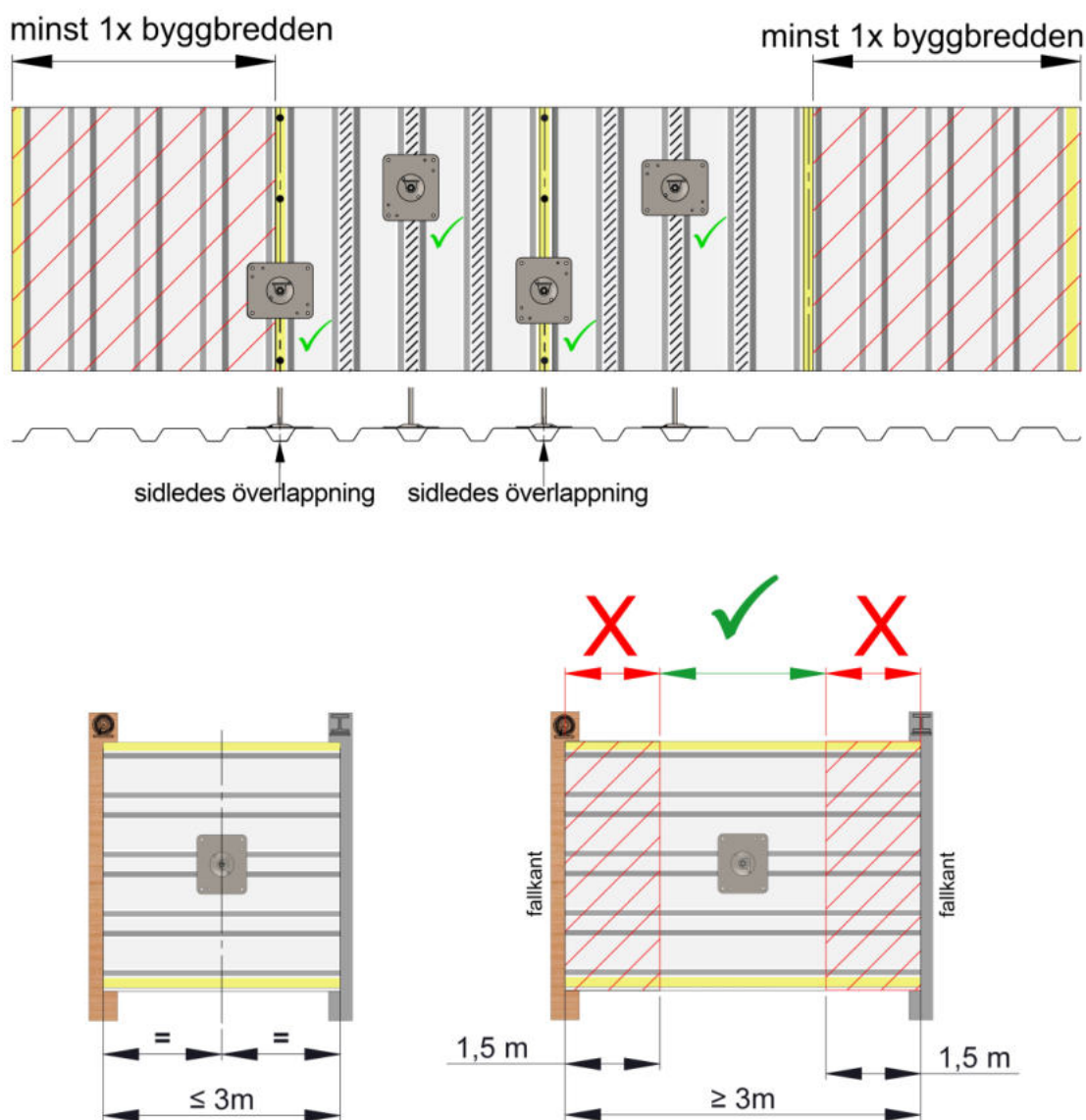
Avstånd till stödet i 1:a fältet
